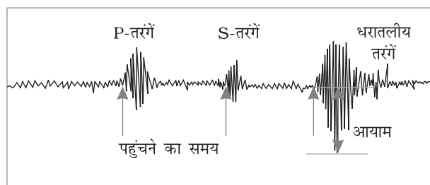
चित्र 3.1 : भूकंप-अभिलेख
