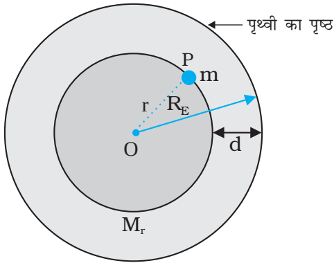
चित्र 7.7 M_E पृथ्वी का द्रव्यमान तथा R_E पृथ्वी की त्रिज्या है, पृथ्वी के पृष्ठ के नीचे d गहराई पर स्थित किसी खान में कोई द्रव्यमान m रखा है। हम पृथ्वी को गोलतः सममित मानते हैं।
